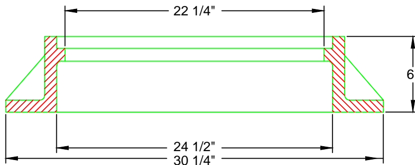
USF 170 MANHOLE RING
